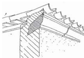
illustration corniche en pierre de taille
