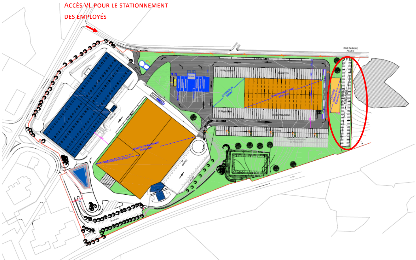
Esquisse du projet de modification de la circulation de l'entreprise DACHSER sur son site au Landreau
